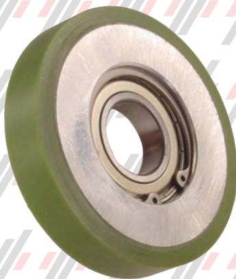
PO290AX1 ROLLER - STEP CHAIN 4" OD RA ESCALATOR
