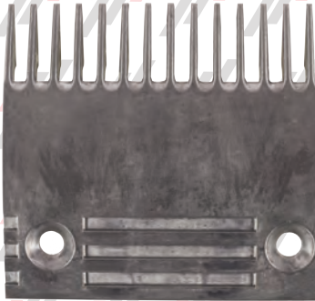
PT1200102 (ALUMINUM) COMBPLATE - LEFT SIDE 14T DONG YANG ESCALATORS
